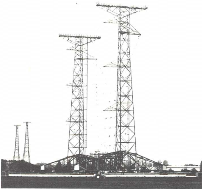
Kurzwellensender Radio Österreich International, Moosbrunn - NÖ, (ORF-Lichtbildstelle)
